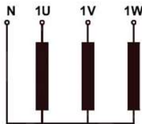
Slika 4.2. Spoj namota trofaznog transformatora u zvijezdu [3]
