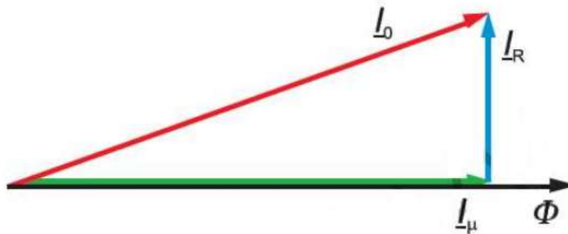
Slika 3.2. Struja magnetiziranja [6]
