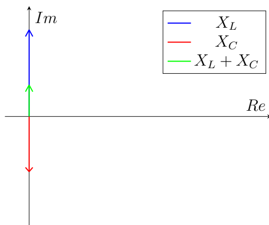
Slika 7.13. Vektori reaktancija u kompleksnoj ravni, izvor: izrada autora
