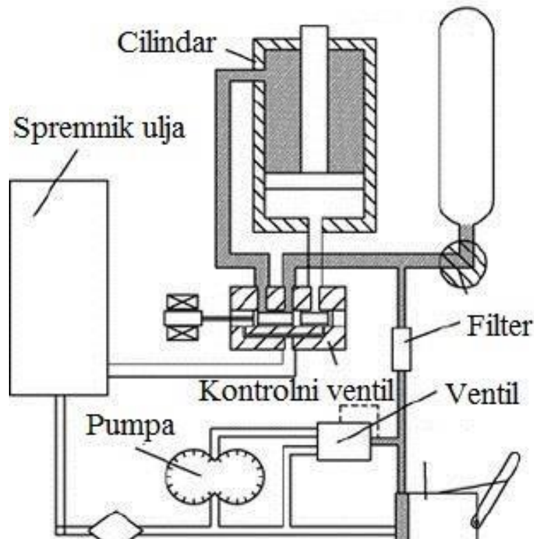
Slika 3.2. Hidraulički mehanizam
