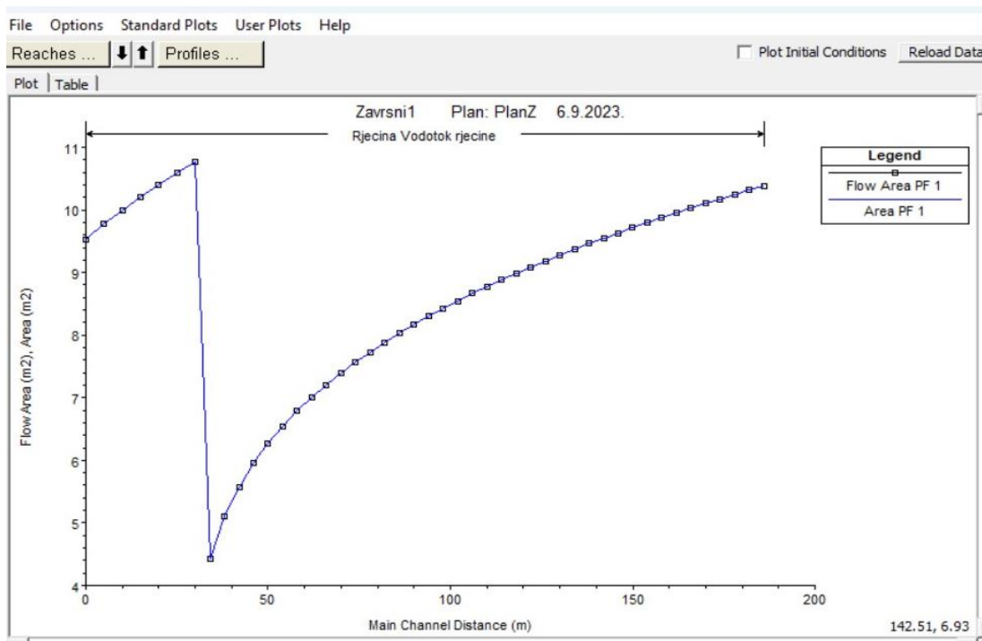
6.8. Graf površine vode kroz odvodni kanal
