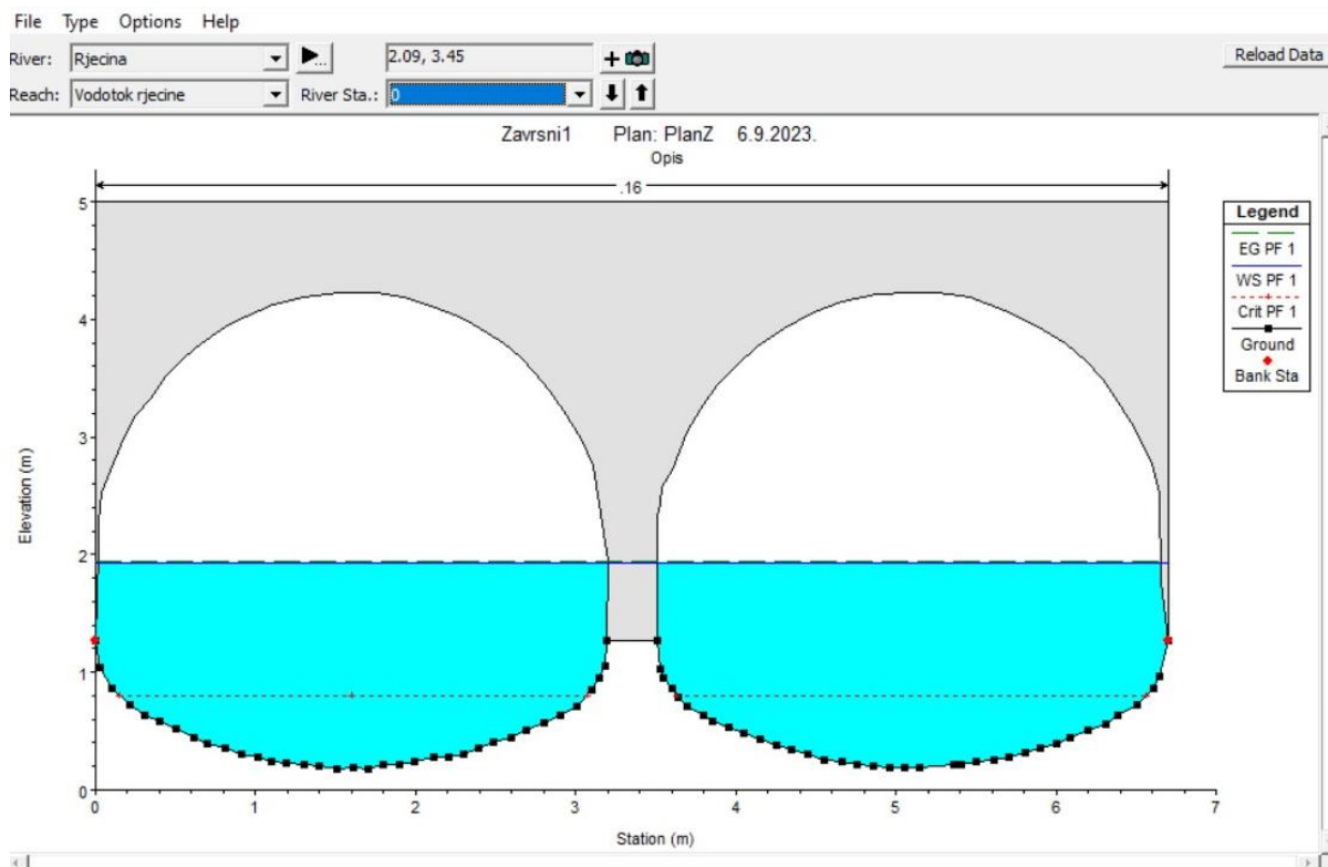
Slika 6.6. Presjek profila 0
