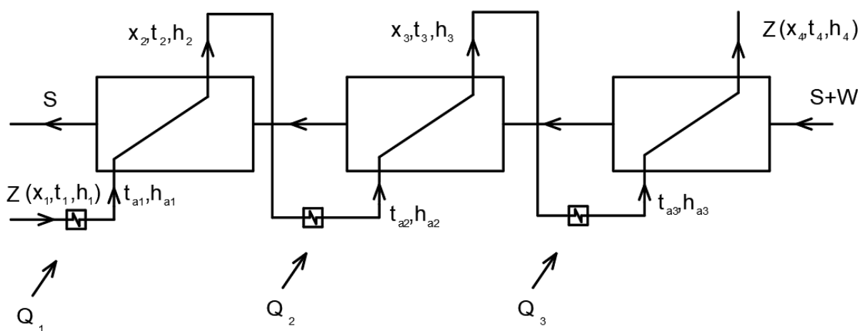
Slika 5.5 Višestepeno sušenje
