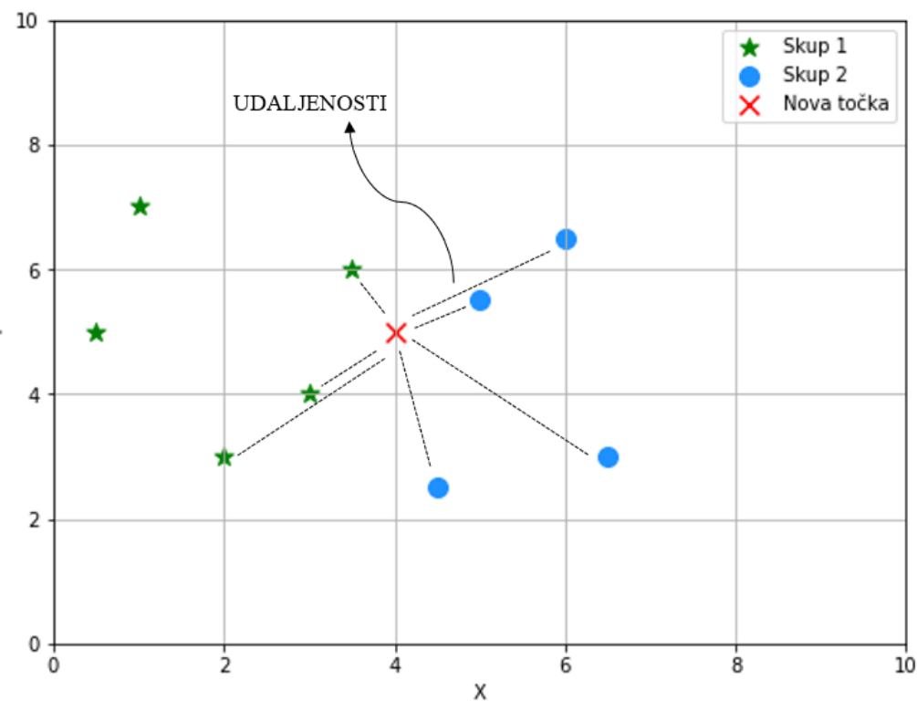
Slika 2.6. kNN algoritam
