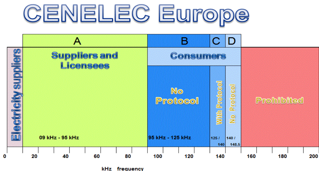
Slika 2.4. Frekvencijska područja PLC-G3 signala [2]
