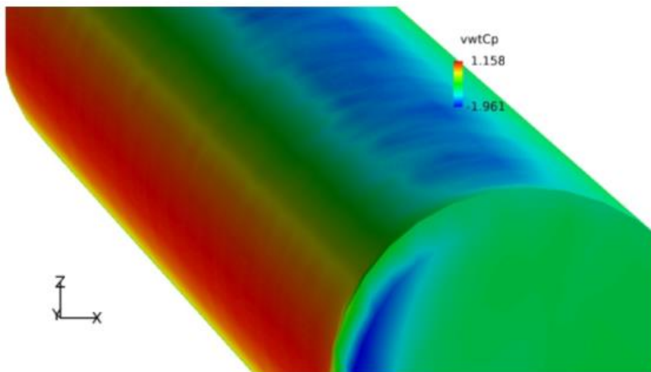
Slika 4.46 : Iznos C_p
