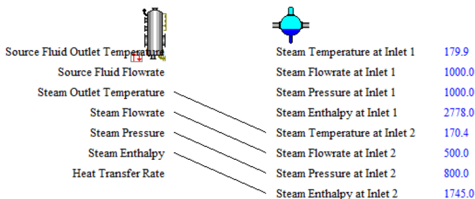
Slika 5.14. Prikaz povezanih podataka za isparivač i parni bubanj
