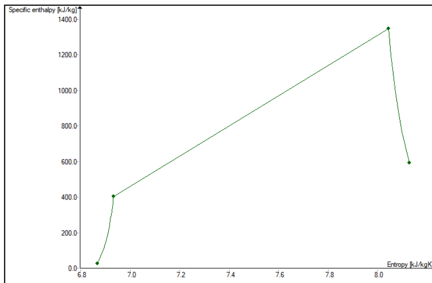
Slika 4.7. h-s dijagram plinskog dijela u izrađena u EBSILON Professional programu
