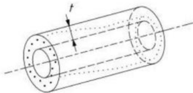
Slika 4.2.1.1. Prikaz toleriranog prostora cilindričnosti elementa [18].
