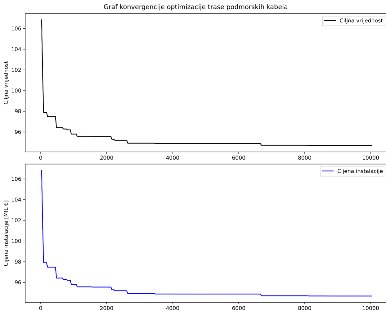
Slika 6-2. Graf konvergencije optimizacije trase podmorskih kabela
