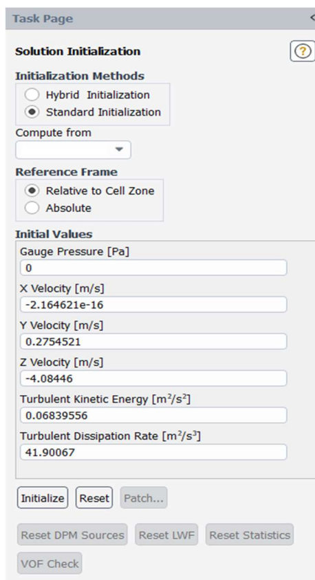
Slika 4.20. Inicijalizacija rješenja
