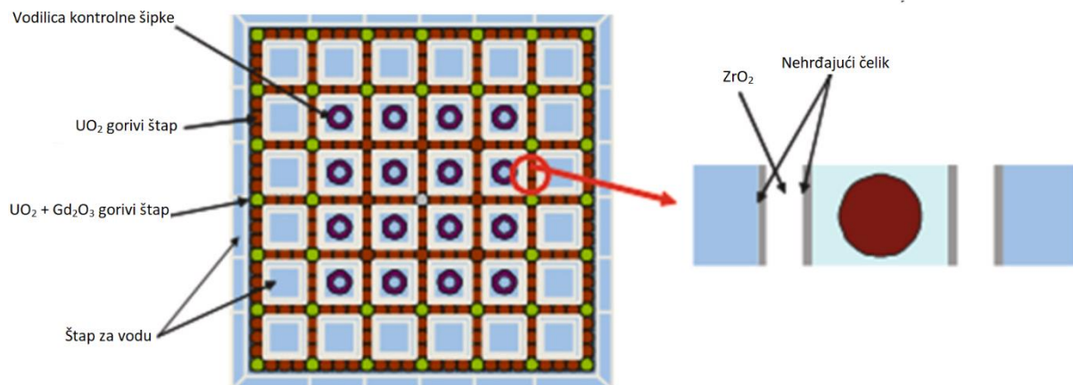
Slika 6.5. Dizajn gorivnog elementa japanskog Super LWR [47]
