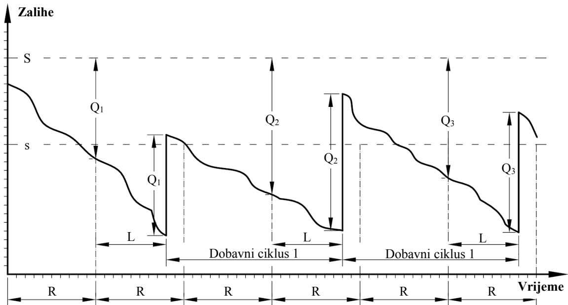
Slika 2.23. (R, s, S) model upravljanja zalihama
