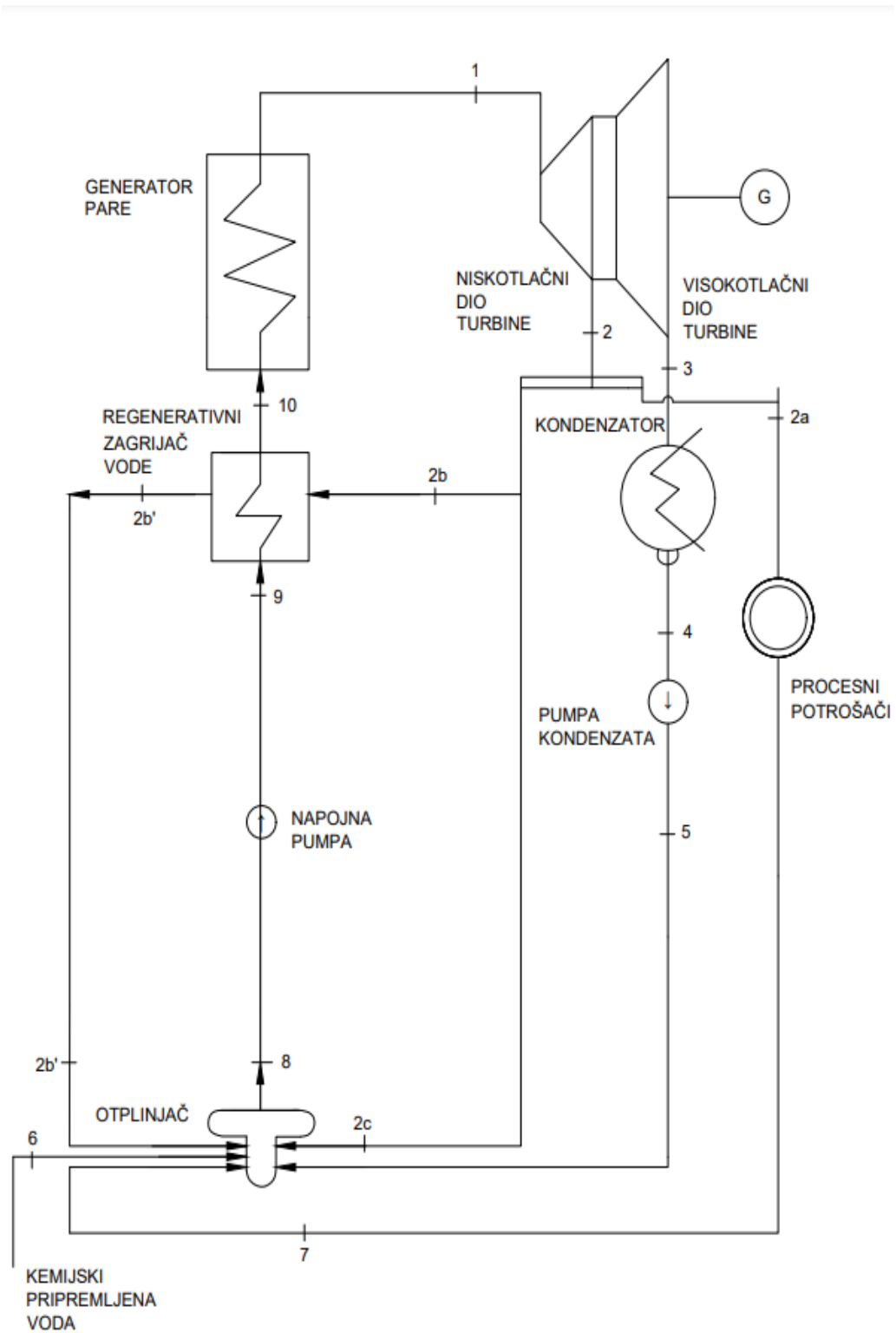
Slika 4.1 Toplinska shema kogeneracijskog postrojenja
