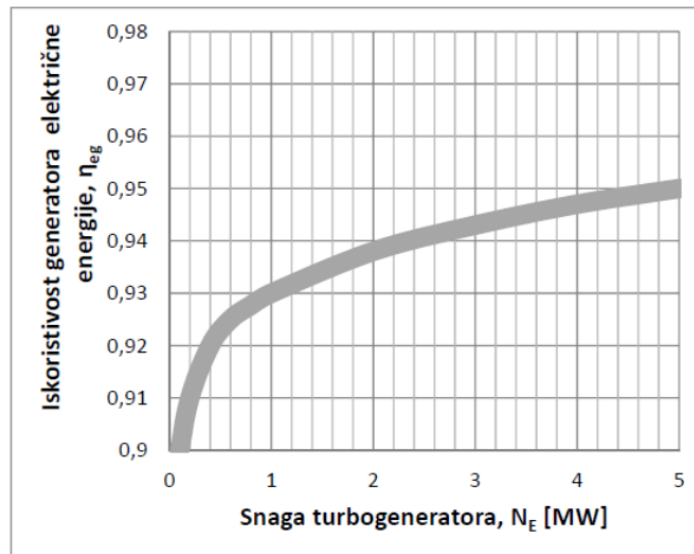
Slika 4.6 Iskoristivost generatora električne energije u zavisnosti od snage [8]
