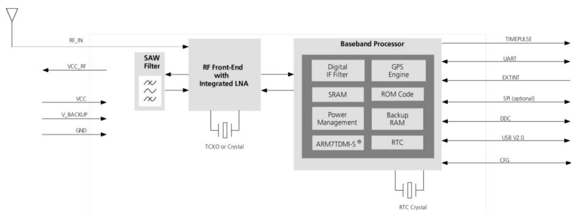
Slika 3.4 Blokovski prikaz NEO-6M GPS modula
