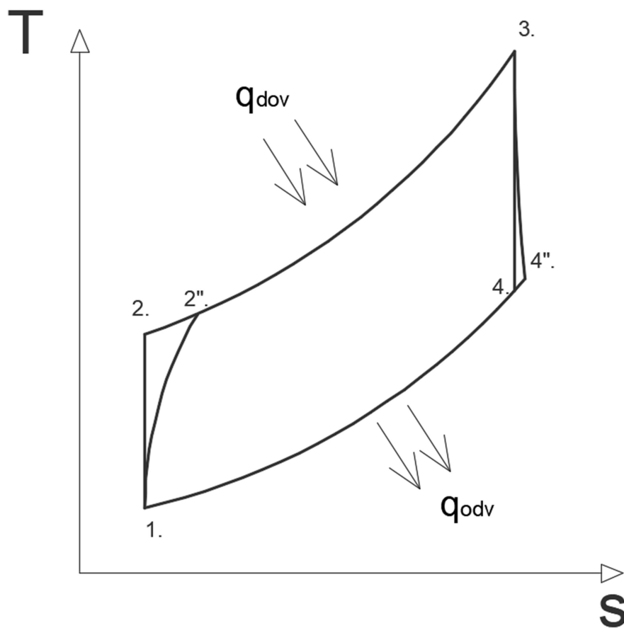
Slika 5.1 T-s dijagram i shema osnovnog zatvorenog sustava
