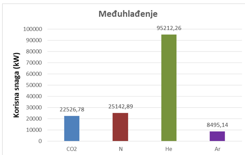
Slika 6.20. Korisna snaga zatvorenog sustava s međuhladnjakom
