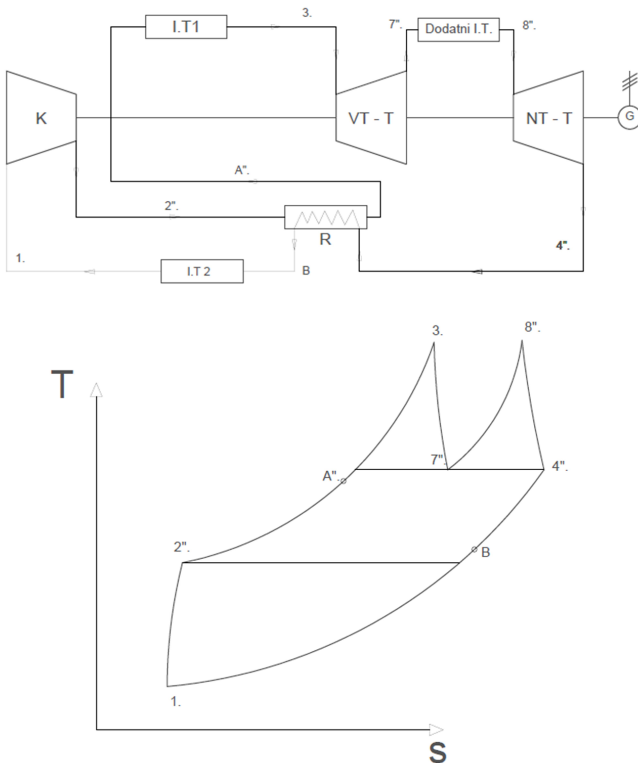
Slika 5.6. Shema i T-s dijagram zatvorenog sustava s dodatnim izmjenjivačem topline i regeneratom
