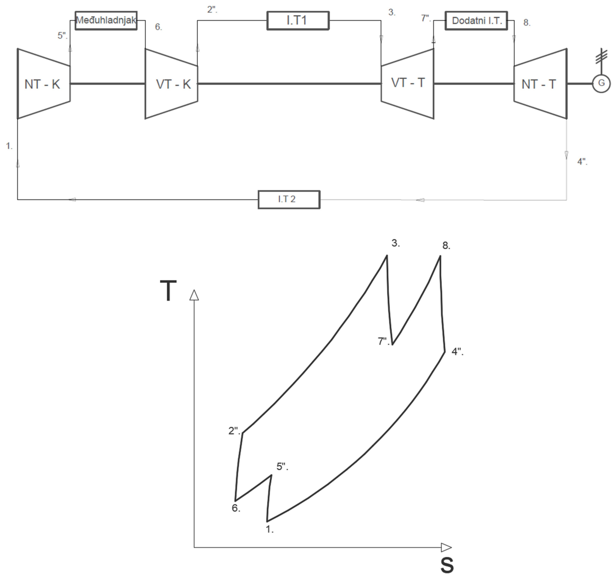
Slika 5.7. Shema i T-s dijagram zatvorenog sustava s međuhladnjakom i dodatnim izmjenjivačem topline
