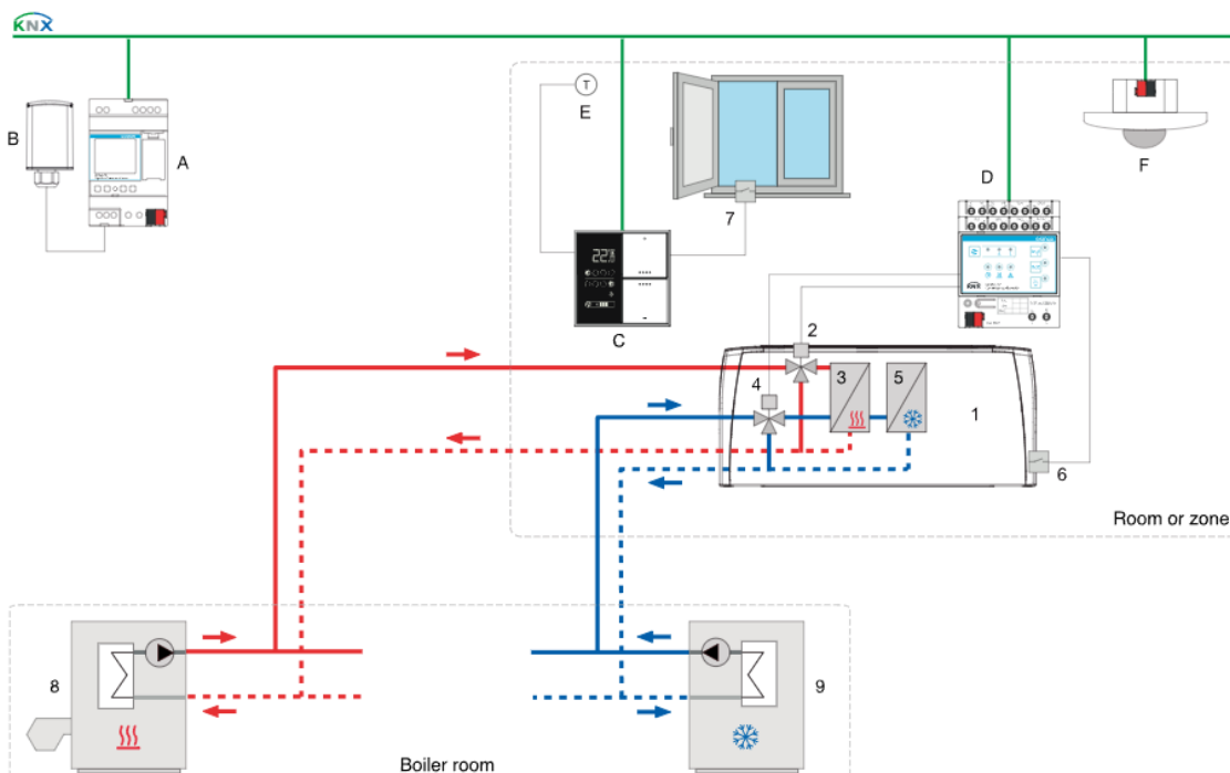
Slika 4.3 - Shema spajanja ventilatorskih konvektora[15]
