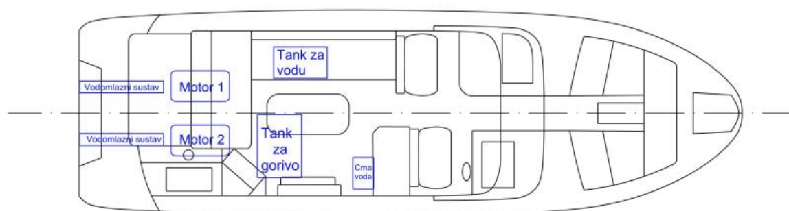
Slika 7.1. Razmještaj glisera sa vodoblaznim pogonom
