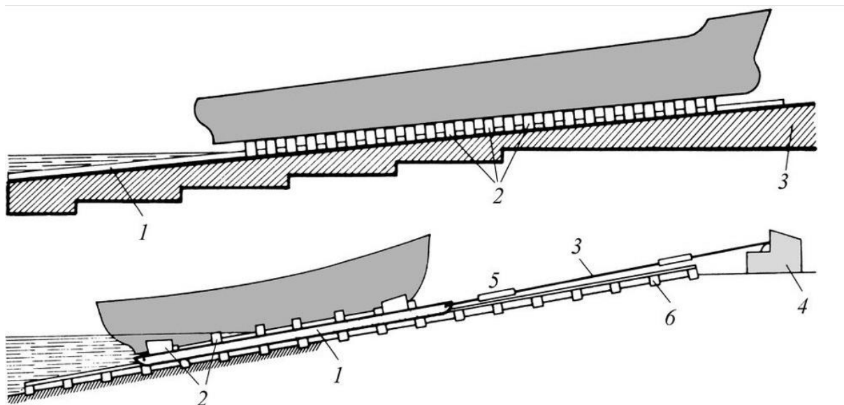
Slika 3.1 Uzdužni navoz: 1)klizna staza, 2)potklada, 3)radna površina (gore); izvlačenje broda na navoz: 1)saonice, 2)kolijevka, 3)uže, 4)vitlo, 5)graničnik, 6)poprečni drveni pragovi (dolje) [6]
