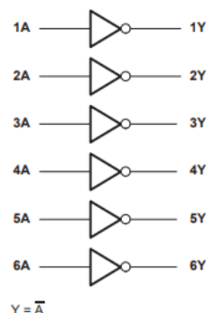
Slika 2.10 SN74LS04N - logički dijagram (Izvor: [8]).
