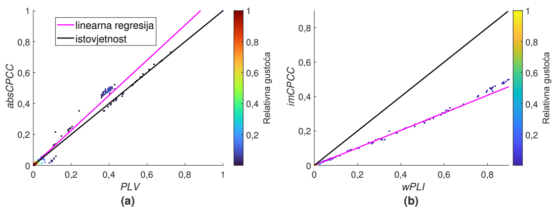
Slika 4.3: Odnosi između mjera statičke funkcionalne povezanosti absCPCC i PLV (a), te imCPCC i wPLI , prikazani dijagramom raspršenja za vrijednosti povezanosti svih parova elektroda na promatranom setu podataka generiranom korištenjem metode generiranja bazirane na Kuramoto modelu koje su predstavljene u [100]. Crni pravac predstavlja idealnu podudarnost rezultata uspoređivanih mjera, dok pravac cijan boje predstavlja linearnu aproksimaciju dobivenih vrijednosti. Točke na slici su obojene prema relativnoj gustoći.
