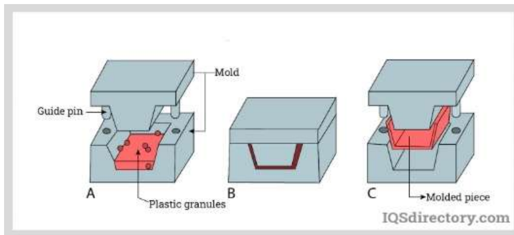
Slika 4.6. Shematski prikaz kompresijskog alata
