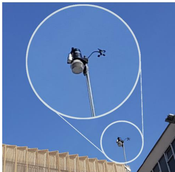
Slika 15: Meteorološka postaja smještena na glavnoj zgradi Tehničkog fakulteta Sveučilišta u Rijeci
