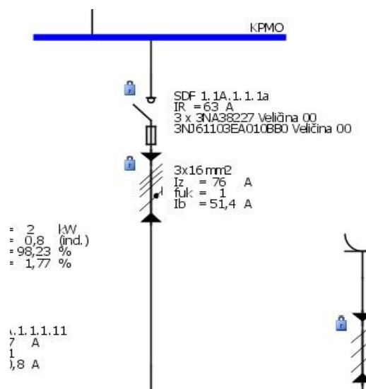
Slika 4.23. Rastalni osigurač na dionici KPMO – RO
