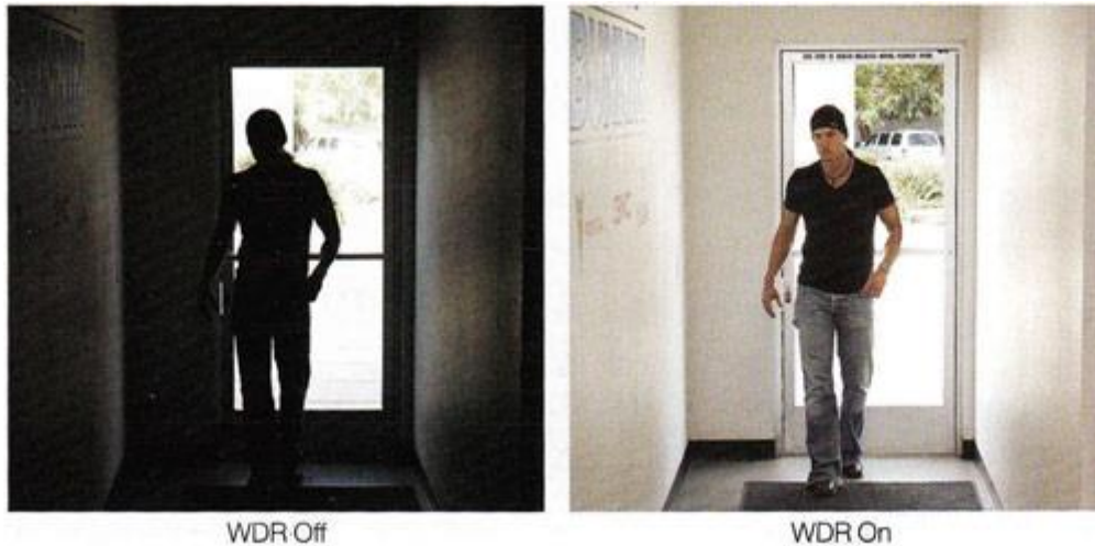
Slika 4.28. WDR [90]
