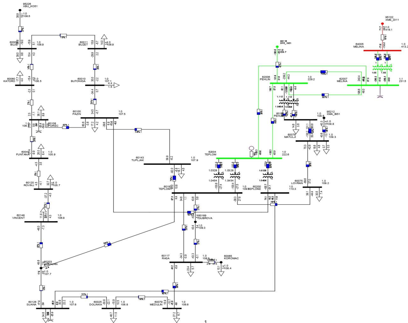
Prilog 10. simulacija Istarskog elektroenergetskog podsustava nakon ugradnje kondenzatorskih baterija u Transformatorske stanice 110 kV Šijana i Poreč za vrijeme nerasploživosti TE Plomin 2 (N-1).
