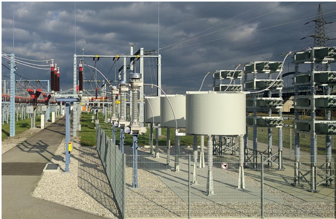
Slika 16. Primjer MSCDn (kondenzatorska baterija i prigušnice) nazivne snage 70 Mvar ugrađene na 115 kV
