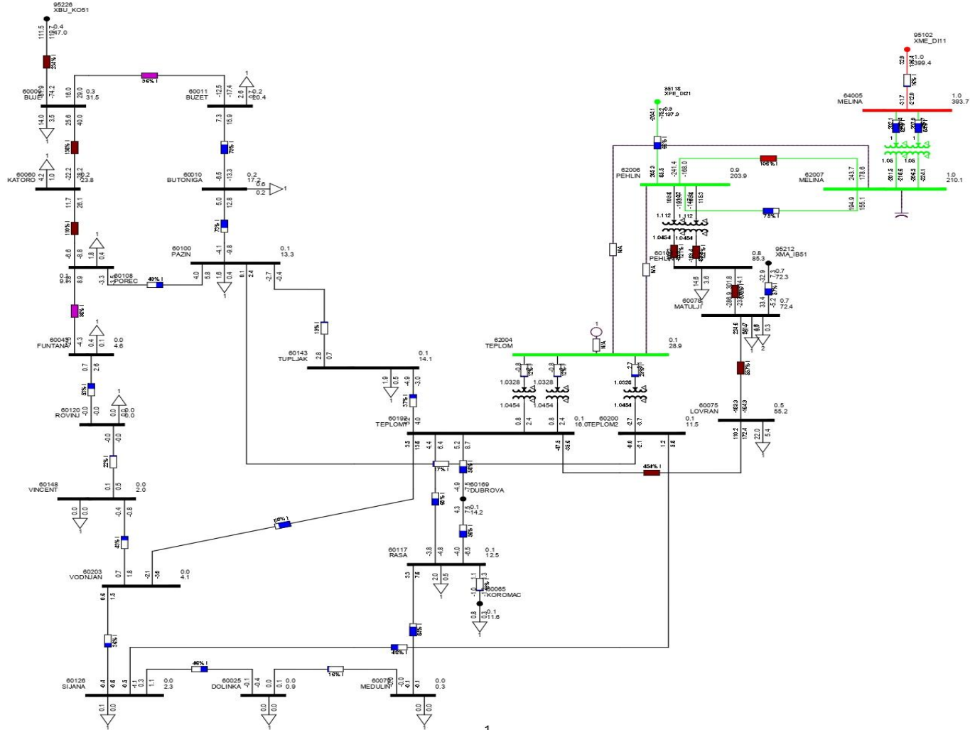
Prilog 3. simulacija trenutnog stanja Istarskog elektroenergetskog podsustava za vrijeme nerasploživosti TE Plomin 2 i dvosistemskog DV 220 kV Melina-Plomin i Pehlin Plomin (N-3).
