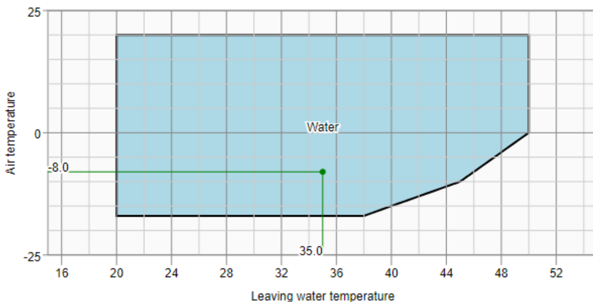
Slika 3.8. Dijagram izlazne temperature vode u odnosu na vanjski zrak kod grijanja [11]
