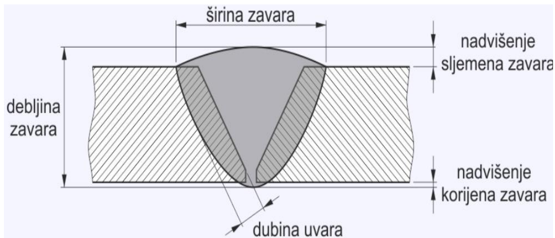
Slika 1.1. 3: Osnovne dimenzije zavora
