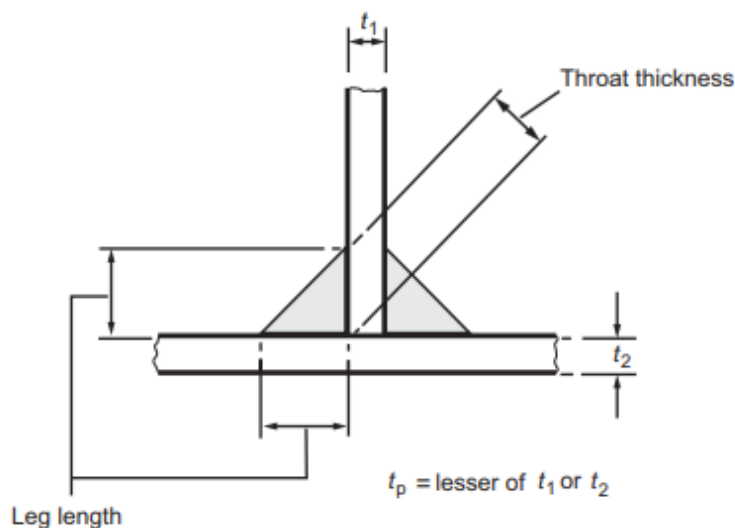
Slika 1.1. 4 Dimenzije zavora prema Lloyd registru
