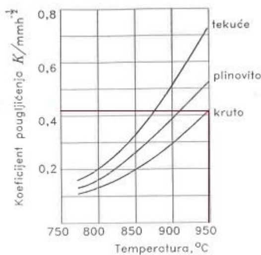
Slika 4.3. Ovisnost koeficijenta pougljičavanja o temperaturi i sredstvu pougljičenja [1]
