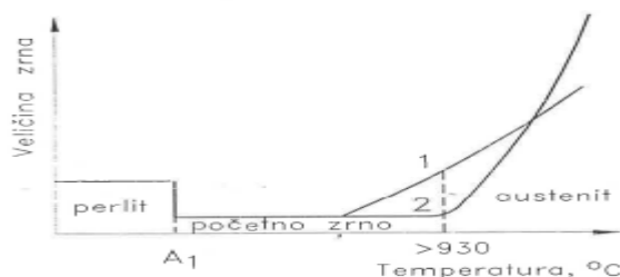
Slika 2.8. Promjena veličine kristalnog zrna austenita ovisno o temperaturi [1]
