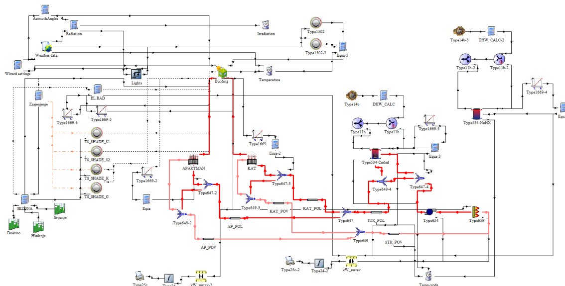
Slika 2.4. Toplinski model
