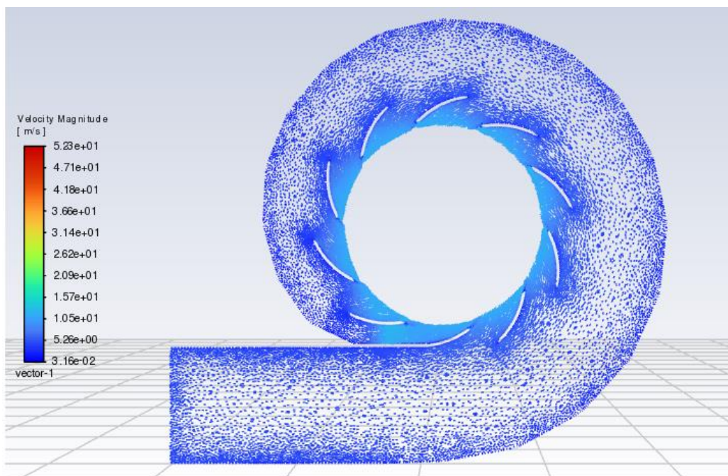
Slika 6.19 Vektori brzina u XZ ravnini za protok od 20 \text{ m}^3/\text{s}
