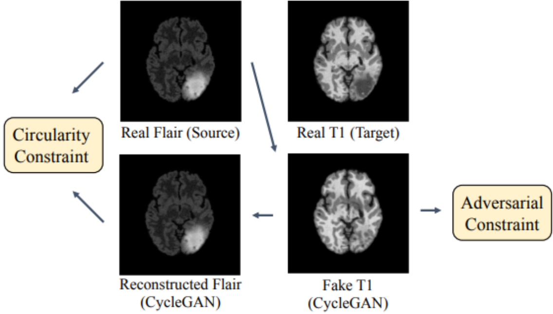
Slika 2.2 Primjer nedostatka dosljednosti ciklusa [9]. Rekonstruirana slika može savršeno odgovarati izvornoj slici (dosljednost ciklusa), dok translahirana slika gubi svojstvo izvorne slike. U ovom primjeru tumor iz izvorne slike ("Real Flair (Source)") se uklanja pri translaciji u ciljanu domenu ("Fake T1").
