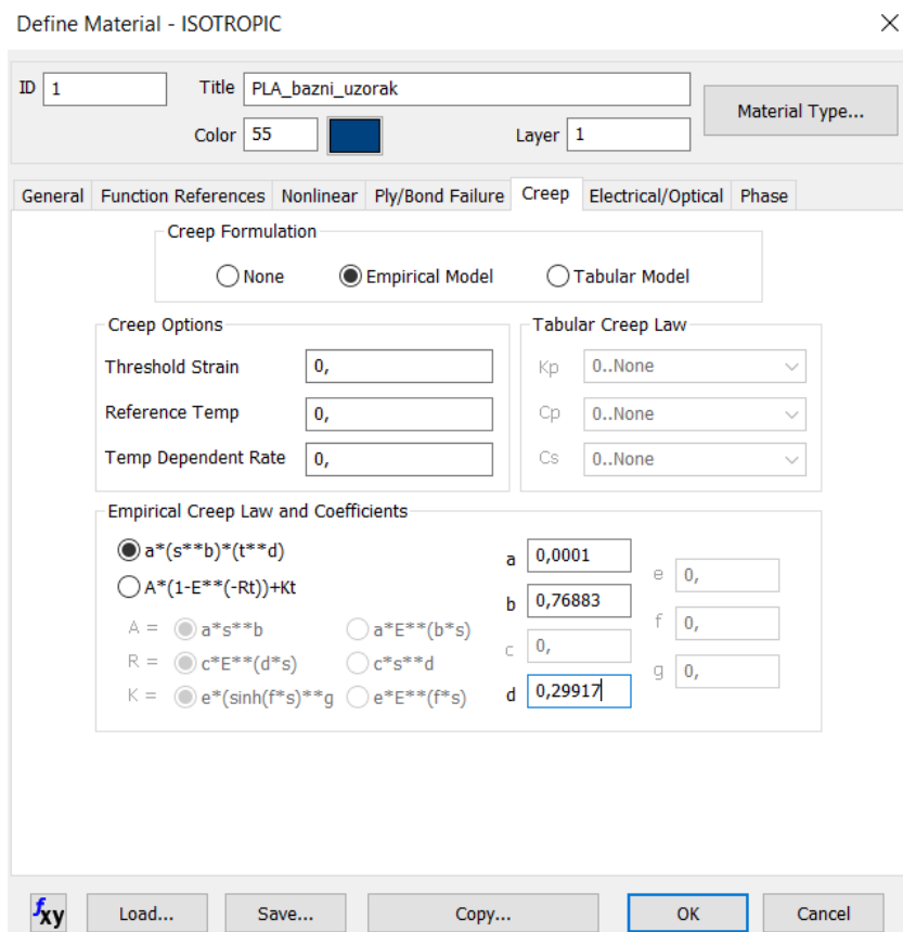
Slika 5.2. Postavke jednadžbe puzanja za materijal
