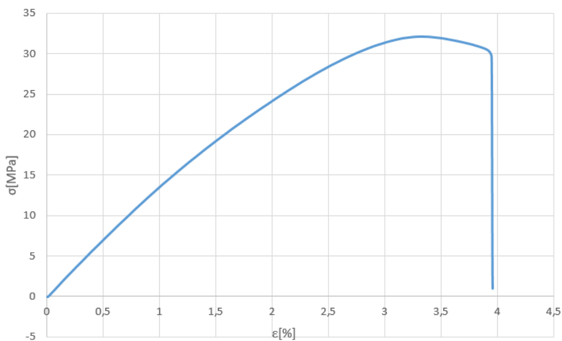
\sigma - \epsilon dijagram (ABS bazni uzorak- serija 2)
