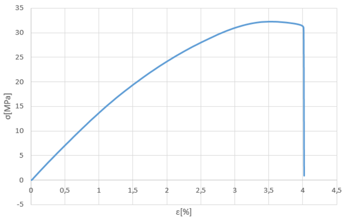
Slika 4.20. \sigma - \epsilon dijagram za ABS uzorak grijan na 60° – serija 1
