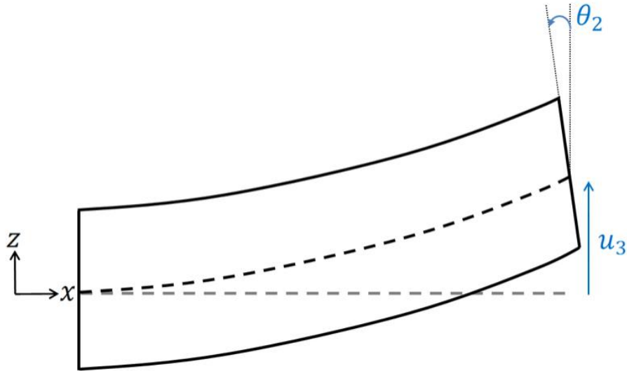
Slika 3.8. Odnosi pomaka i rotacije elementa u xz ravnini
