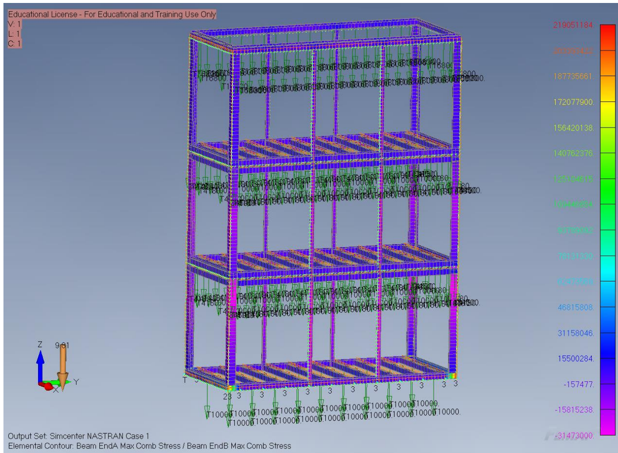
Slika 8.8. Maksimalna kombinirana napreznanja analize tri kontejnera
