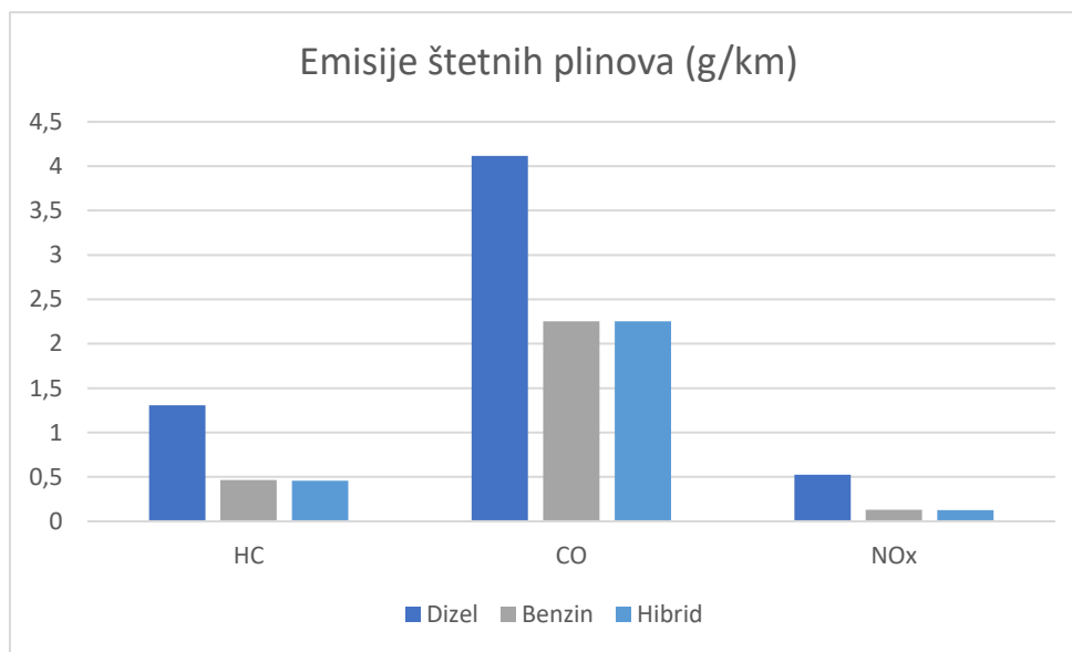
Slika 4.3. Usporedba emisije štetnih plinova za gradsku vožnju
