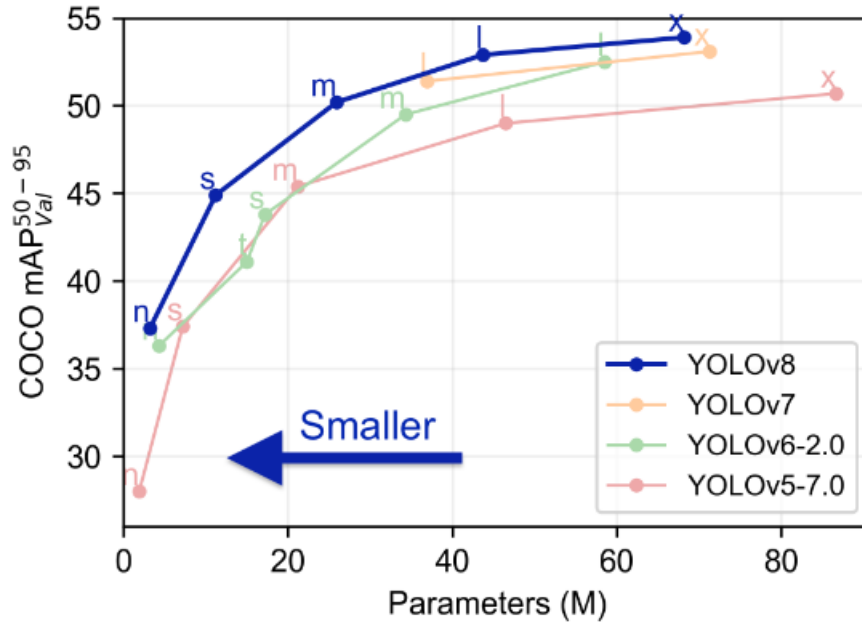
Slika 3.3 Usporedba broja parametara različitih YOLO modela.[2] Os apscisa prikazuje broj parametara, dok os ordinata prikazuje srednju prosječnu preciznost korištenjem COCO protokola evaluacije na COCO skupu podataka. Svaka točka predstavlja drugačiji modalitet rada određenog YOLO modela.
