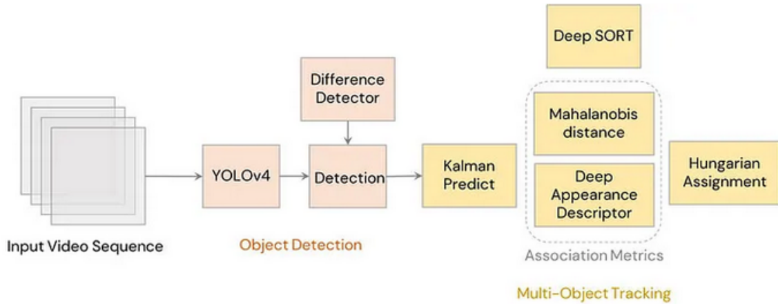
Slika 5.2 Prikaz ulaza i konfiguracije Deep SORT algoritma.[21]
