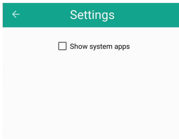
Slika 3.21 Postavke aplikacije
