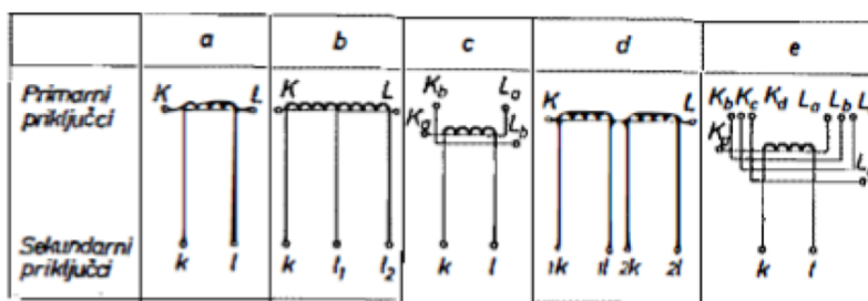
Slika 5: Označavanje stezaljki strujnog transformatora. [1]
