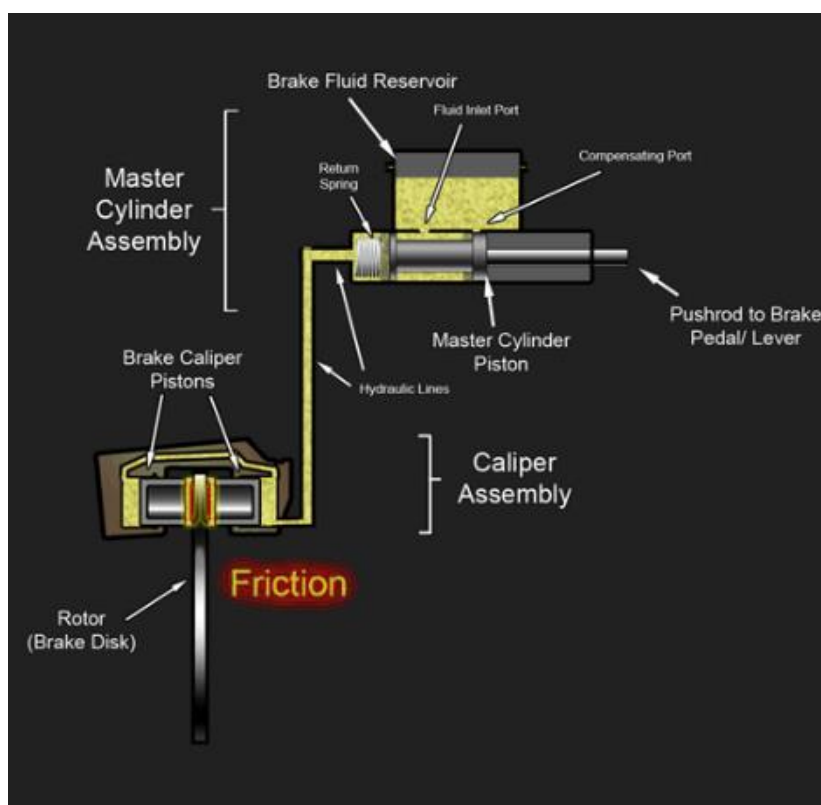
Slika 4.23. Hidraulički sustav za vrijeme kočenja [18]
