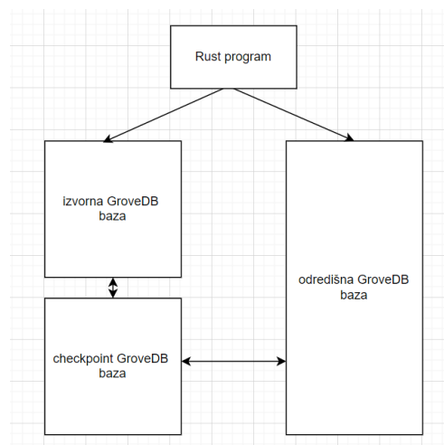
Slika 3.11 GroveDB replikacija
