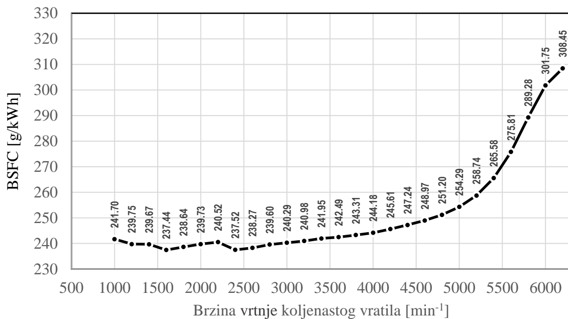
Slika 4.15. Krivulja BSFC – tri ventila, promjeri određeni programom
