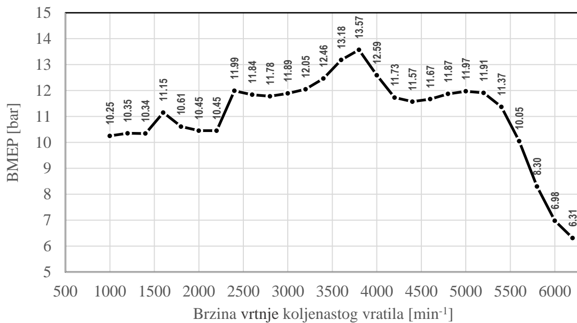
Slika 4.16. Krivulja BMEP – tri ventila, promjeri određeni programom
