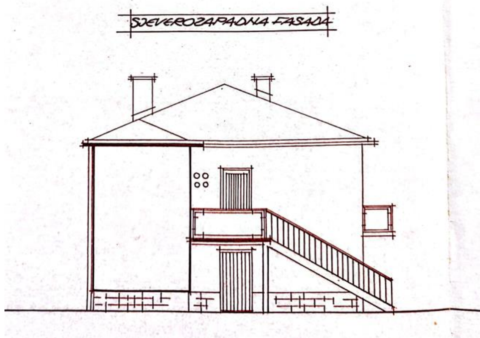
Slika 2.7. Sjeverozapadna fasada
