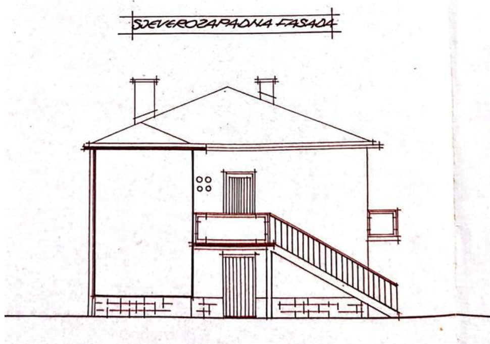
Slika 2.7. Sjeverozapadna fasada
