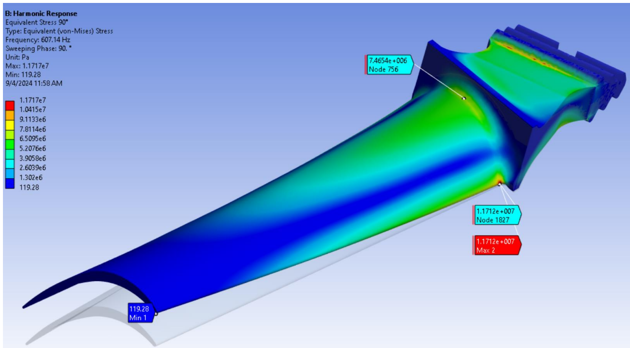
Slika 5.5 Ekvivalentno naprežanje
