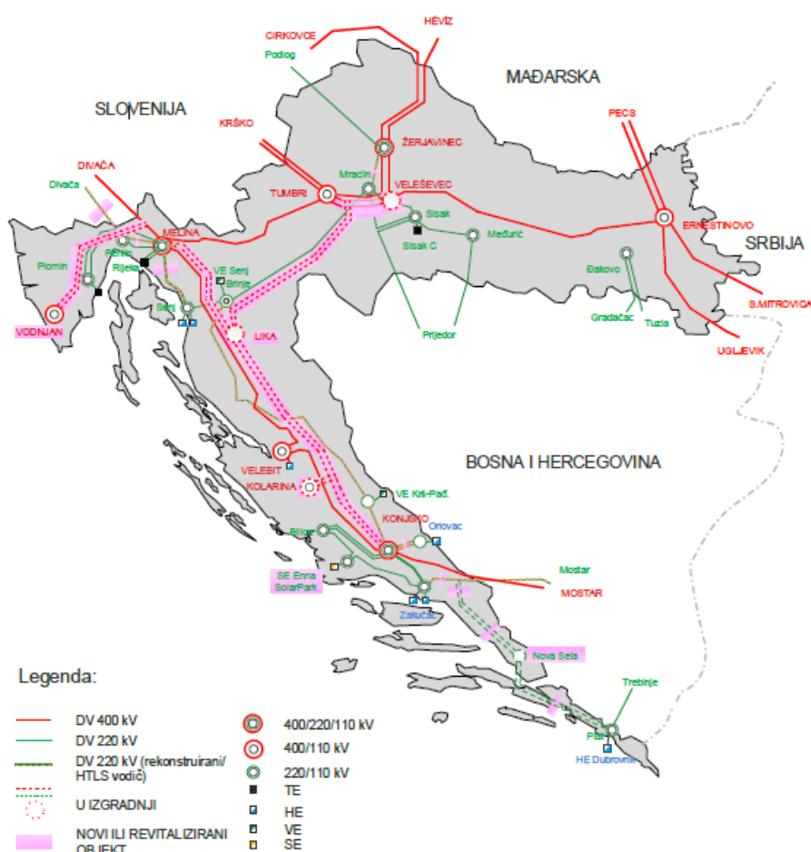
Slika 2.3. Prikaz konfiguracije prijenosne mreže krajem 2032. godine [9]
