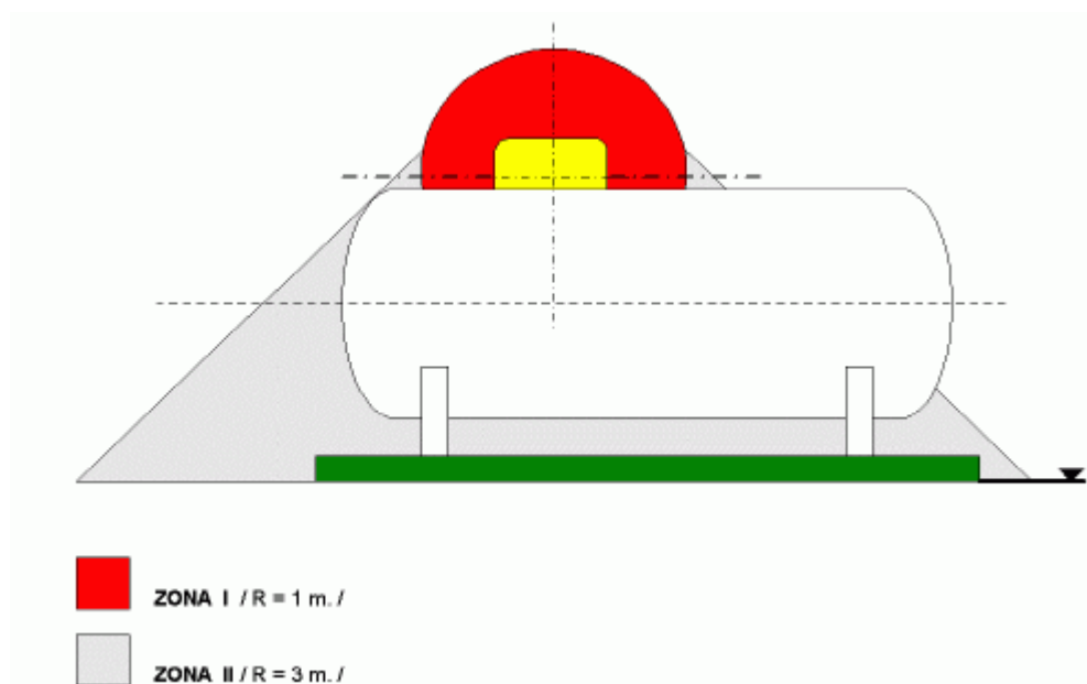
Slika 2.1: Zone opasnosti [1]
