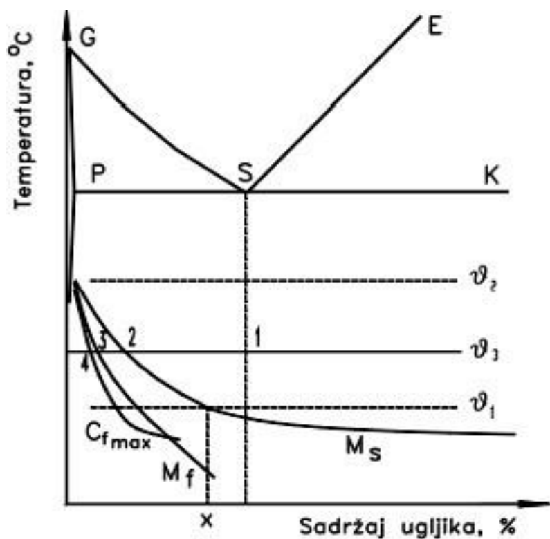
Slika 2.11. Shematski prikaz područja bainitne pretvorbe
