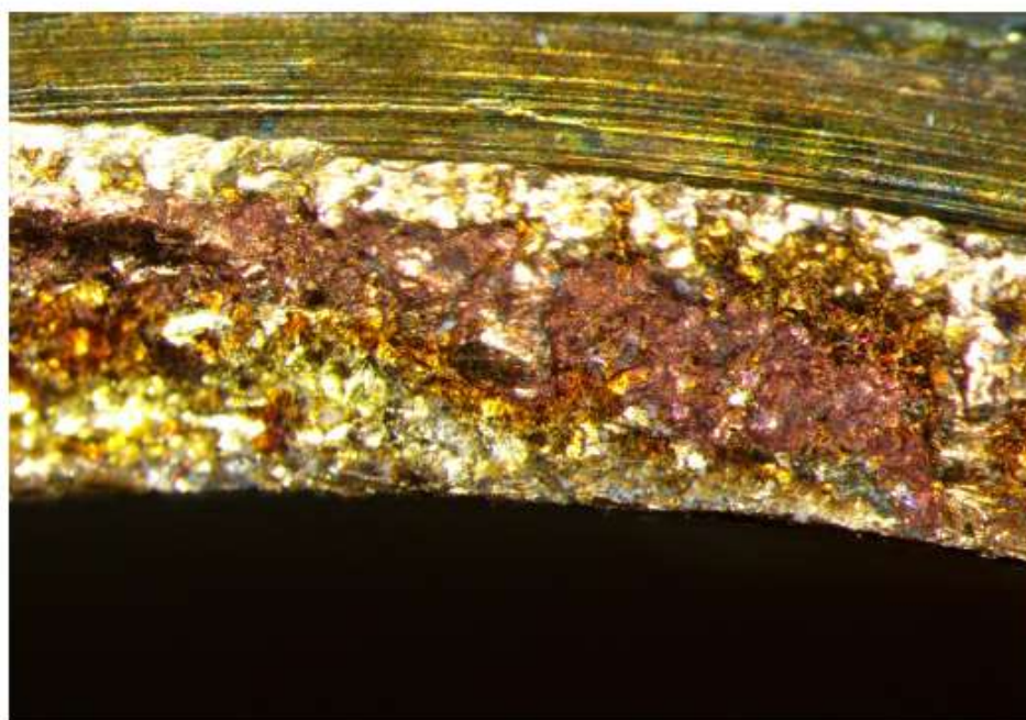
Slika 3.18 Primjer decinkacije uložka slavine [17]
