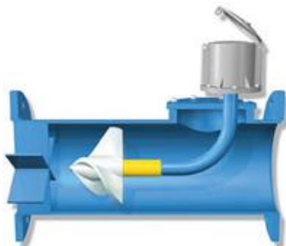
Slika 3.3. Prikaz propelernog protokomjera [29]
