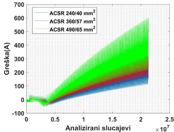
Slika 8. Izračunate razlike između proračuna stacionarnog DTO-a razmatranih ACSR vodiča metodologijama Cigre 601 i IEEE 738
